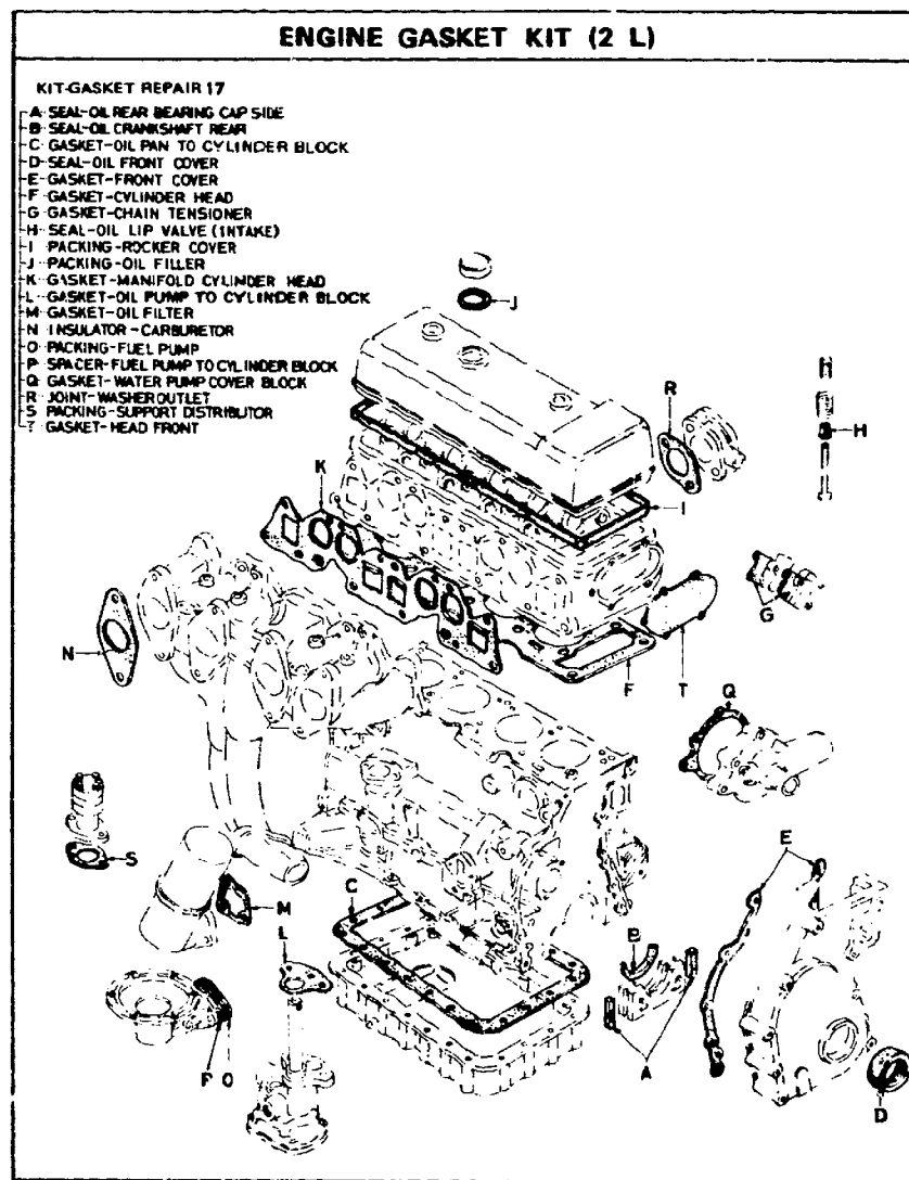
FIG. 0A-3 D6 NISSAN MOTOR CO., LTD.
