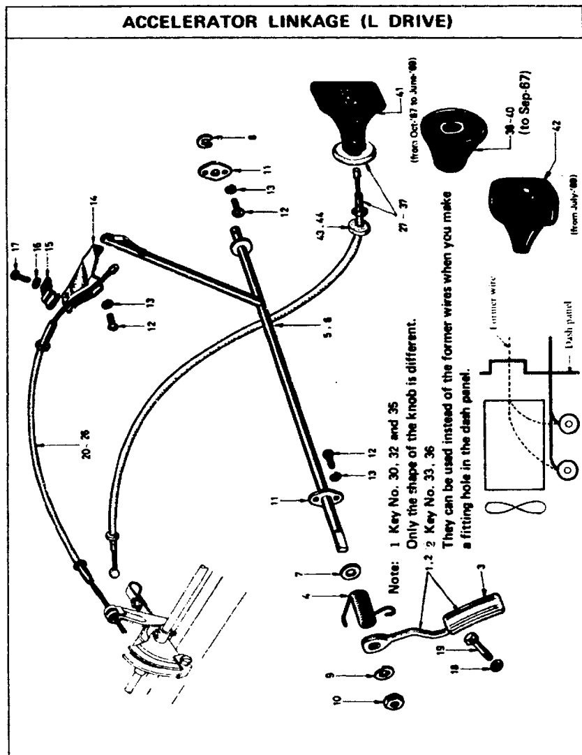
FIG. 13 15 NISSAN MOTOR CO., LTD.
