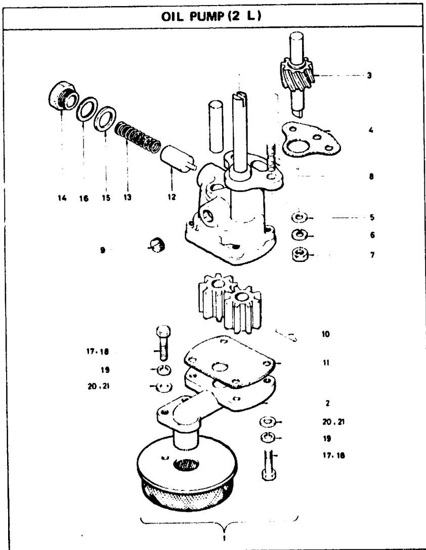
FIG. 6A F15 NISSAN MOTOR CO., LTD.
