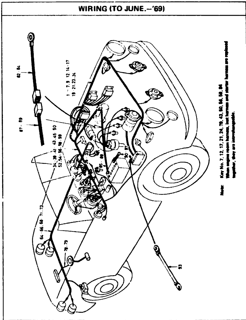
FIG. 22-1 L9 NISSAN MOTOR CO., LTD.
