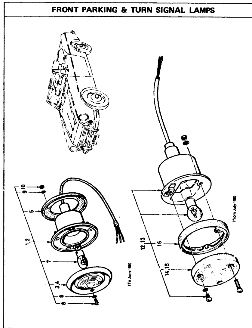
FIG. 26 N2 NISSAN MOTOR CO., LTD.
