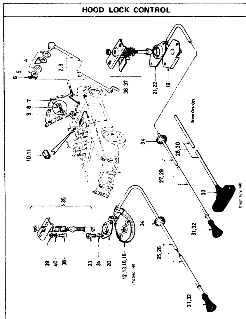
FIG. 55A J8 NISSAN MOTOR CO., LTD.
